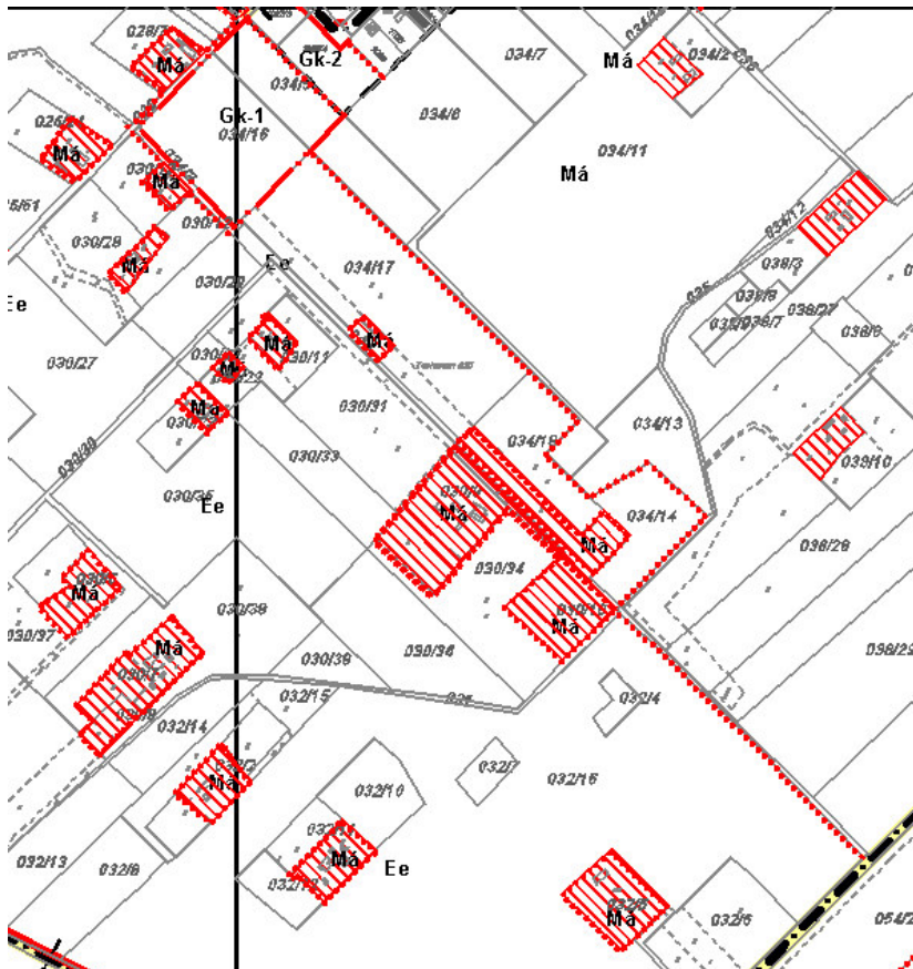
3. tervrészlet
